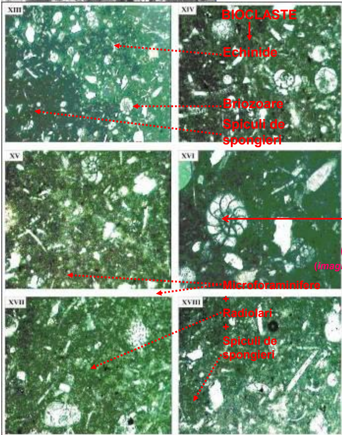
Bioclaste în calcare bioclastice (Flișul extern carpatic) (imagine la microscop din Calcarele de Doamna)
